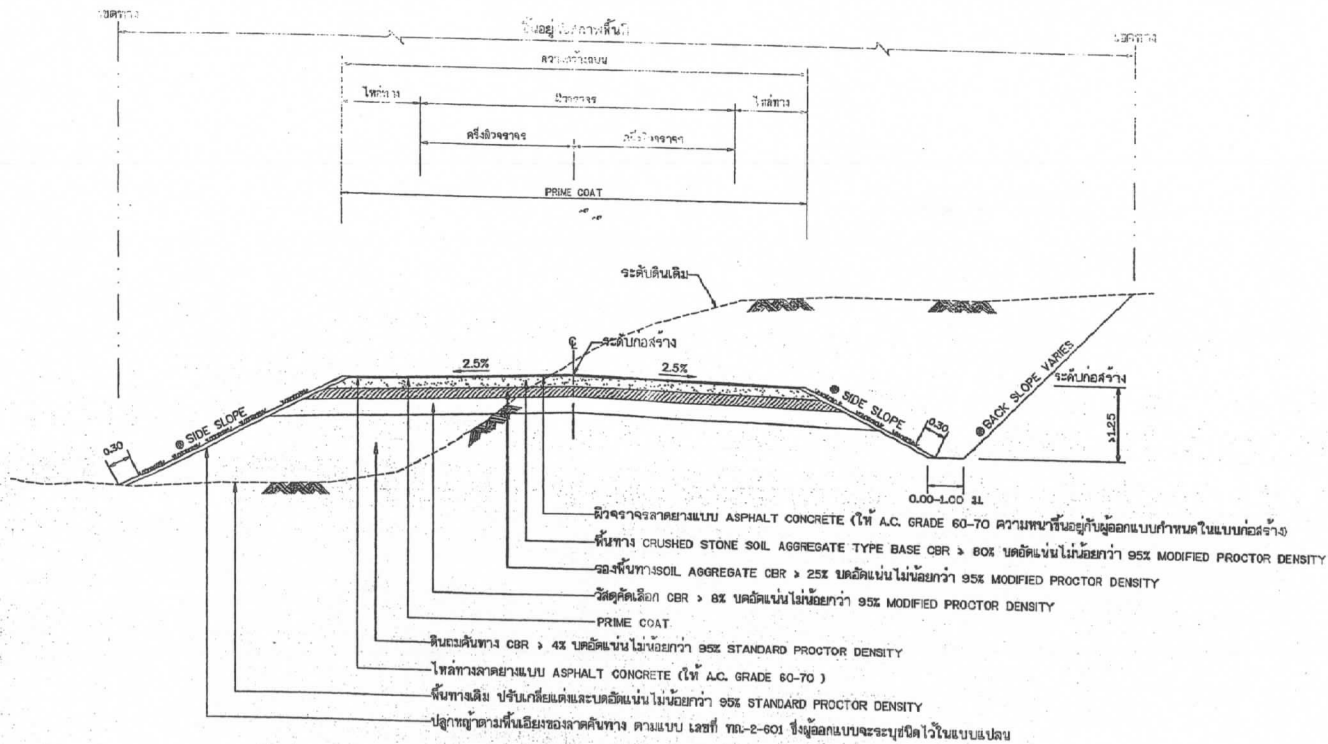
รูปตัดแสดงโครงสร้างถนนดินตัด ดินถมและคลุมสุมบิวส์
