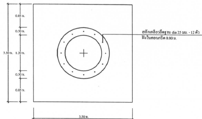
แบบขยายฐานรากหอดังสูง (แบบฐานแต่) มาตรฐาน 1 : 50
