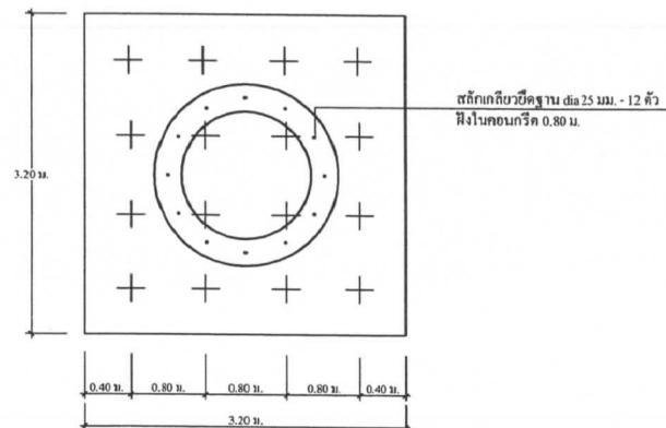
แบบขยายฐานรากหอดังสูง (แบบเสริม) มาตรฐาน 1 : 50
