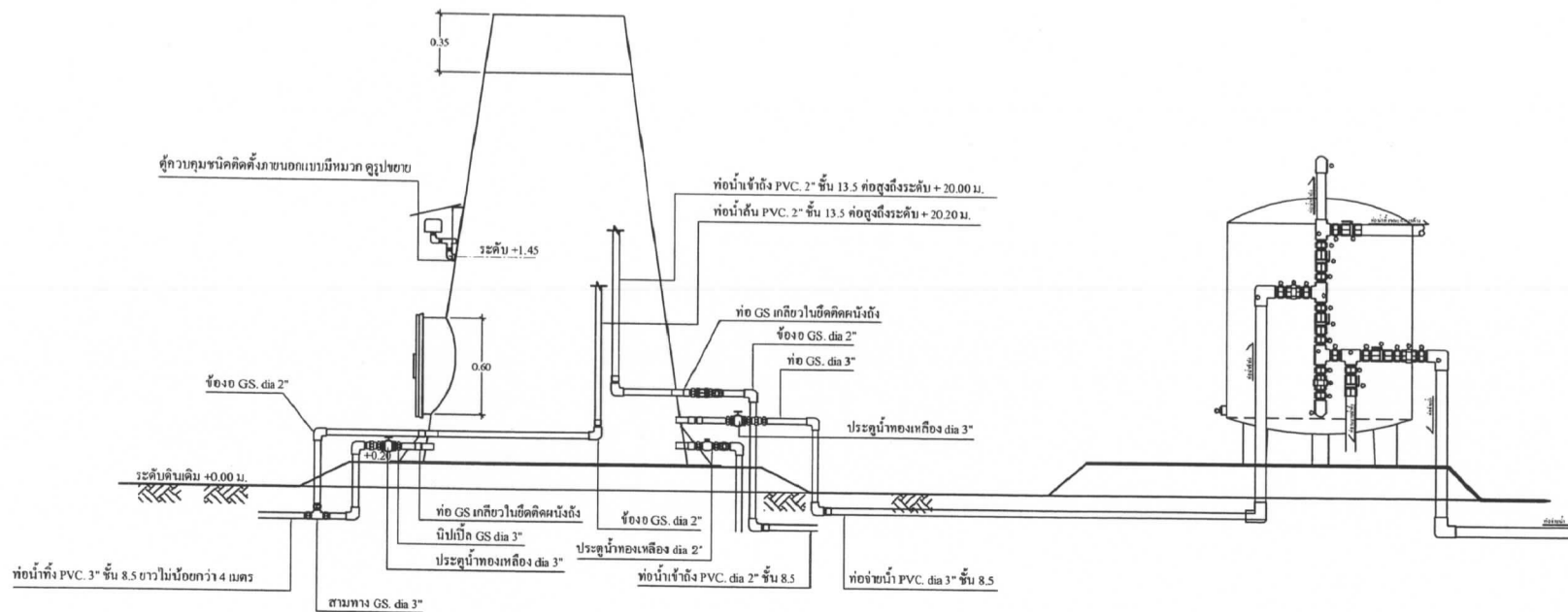
แบบการติดตั้งถังกรองน้ำเข้ากับห้องสูง มาตราส่วน 1 : 25
