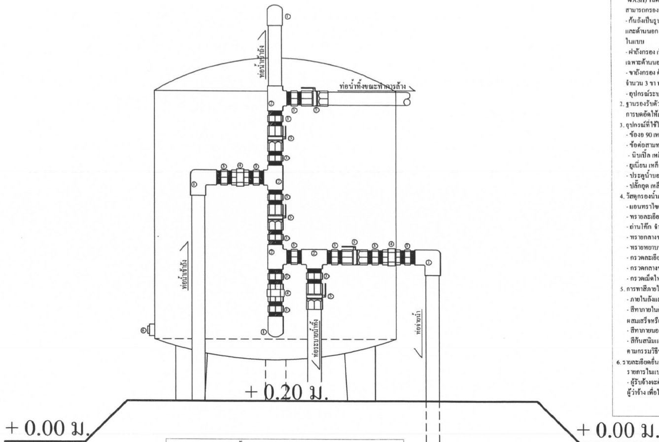
แบบขยายรูปด้านตั้งและอุปกรณ์ภายนอก ถึงกรงสนิมเหล็ก มาตราส่วน 1 : 10
