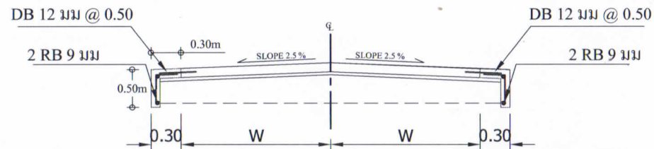
รูปตัดโครงสร้าง คานป้องกันการกัดเซาะขอบถนน
