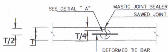
LONGITUDINAL JOINT
