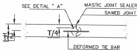
LONGITUDINAL JOINT
