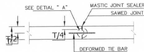
LONGITUDINAL JOINT
