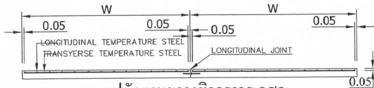
รูปตัดตามขวางผิวจราจร คสส.
