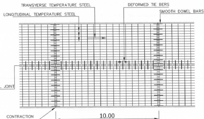
แปลนแสดงการเสริมเหล็กถนน ค.ส.ค.
