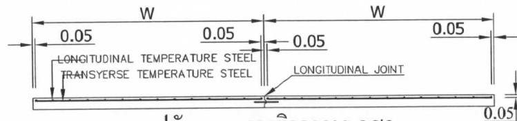
รูปตัดตามขวางผิวจราจร คสค.
