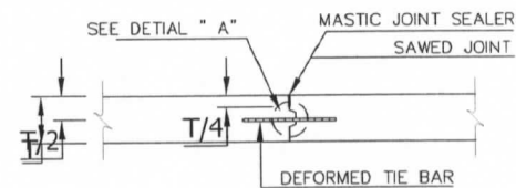
LONGITUDINAL JOINT
